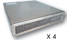
Dim. générateur : 312 x 330 x 68 mm
